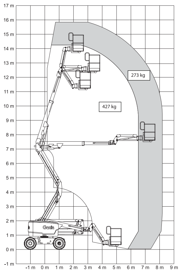
Arbajdsområdediagram for Z-45 XC med flybeskyttelse
